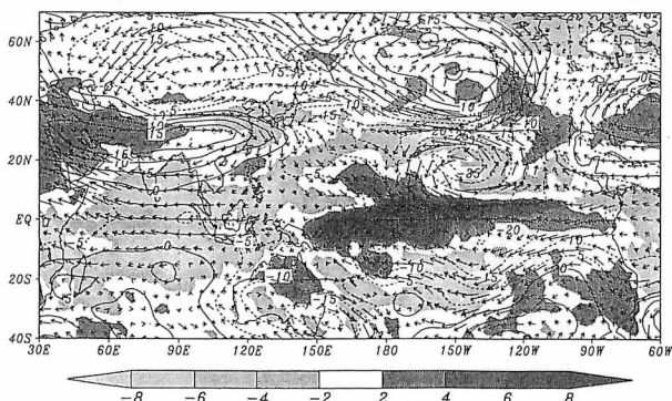
図10 モンスーンに先行する冬季における層厚 (200 hPa - 500hPa), 200 hPa 風ベクトル, OLR のそれぞれ偏差の合成図 a) 弱モンスーン年(1983, 1987, 1992年), b) 強モンスーン年(1984, 1985, 1990年), 等値線間隔は 5 m, ベクトルの単位は 8 m/s, 陰影部は OLR の偏差で単位は W/m^2 .
