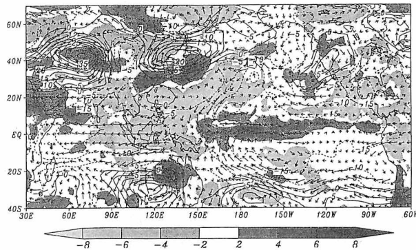
図15 図14と同様、ただしデータはECMWF
